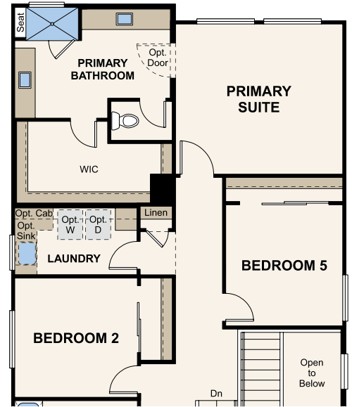
OPT. BEDROOM 5
